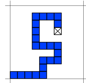
Autres algorithmes : tentatives de pavage aléatoire
