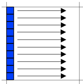
Algorithme optimal
